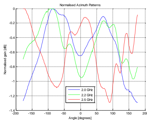
Azimuth (H-plane)
